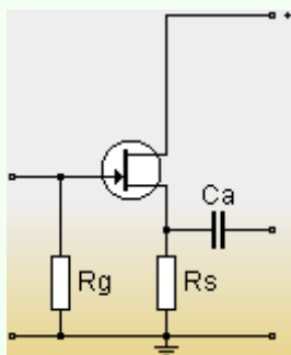
Abbildung 2-1: Einfacher FET-Impedanzwandler
