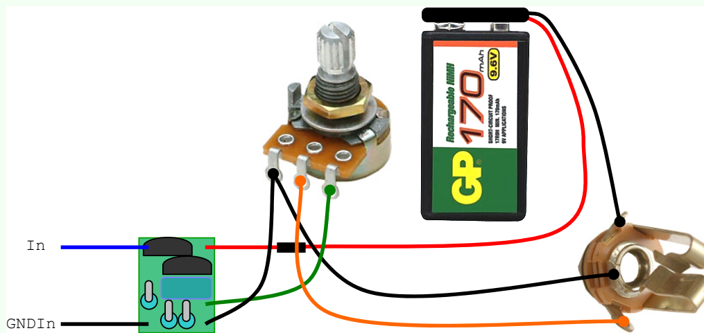
Abbildung 3-3: SB-1-C1 mit Lautstärkeeinsteller vor der Ausgangsbuchse
