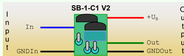
Abbildung 3-1: Die Platine des SB-1-C1
