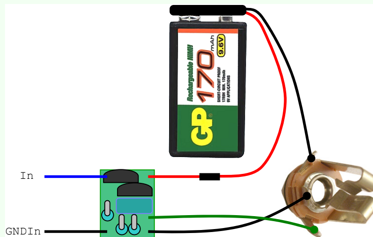
Abbildung 3-2: SB-1-D1 direkt vor der Ausgangsbuchse
