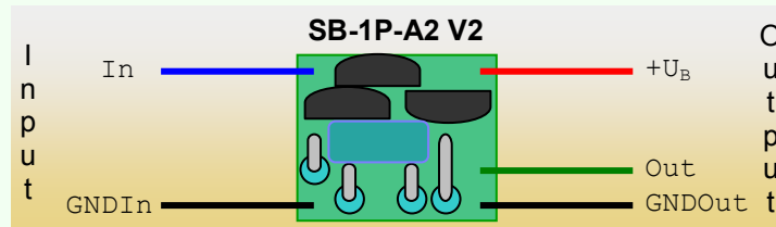
Abbildung 3-1: Die Platine des SB-1P-A2
