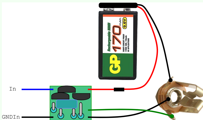
Abbildung 3-2: SB-1P-B2 direkt vor der Ausgangsbuchse
