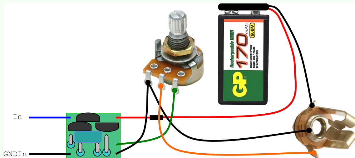
Abbildung 3-3: SB-1P-B2 mit Lautstärkeinsteller vor der Ausgangsbuchse
