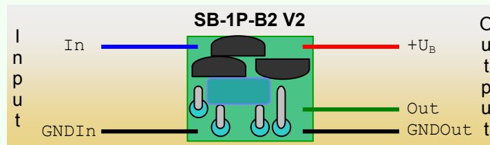
Abbildung 3-1: Die Platine des SB-1P-B2
