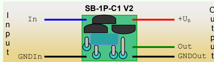
Abbildung 3-1: Die Platine des SB-1P-C1
