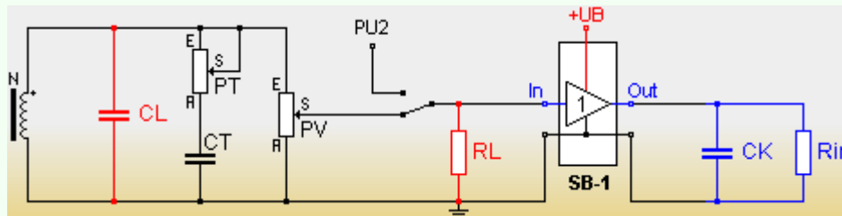
Abbildung 6-3: Paula-Setup mit Impedanzwandler
