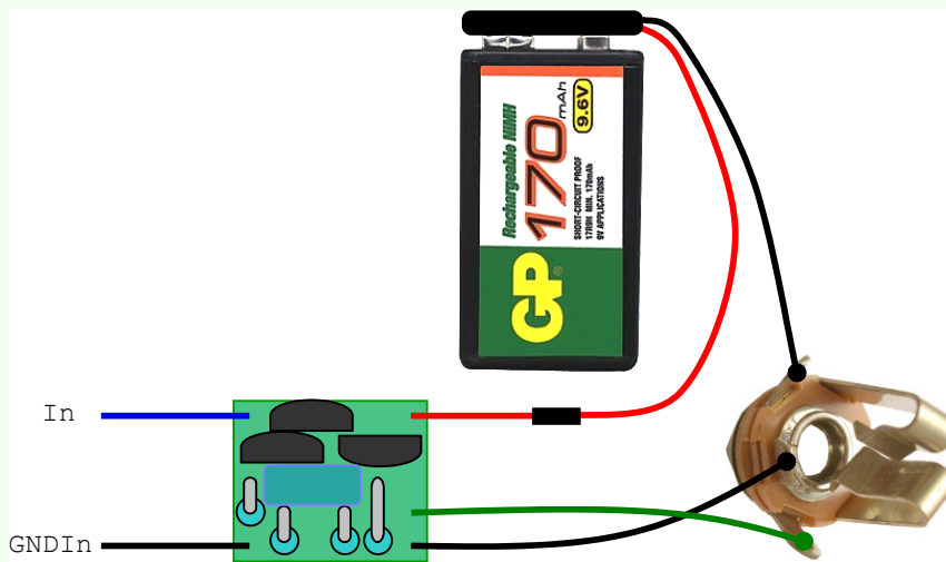
Abbildung 3-2: SB-1P-D1 direkt vor der Ausgangsbuchse
