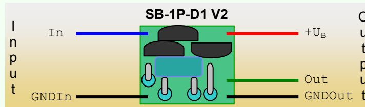
Abbildung 3-1: Die Platine des SB-1P-D1
