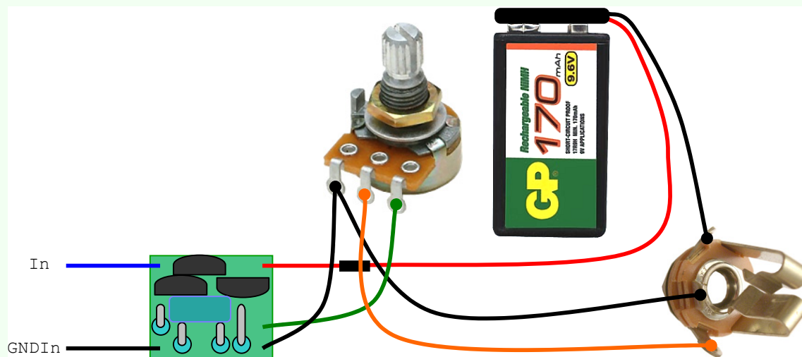
Abbildung 3-3: SB-1P-D1 mit Lautstärkeinsteller vor der Ausgangsbuchse
