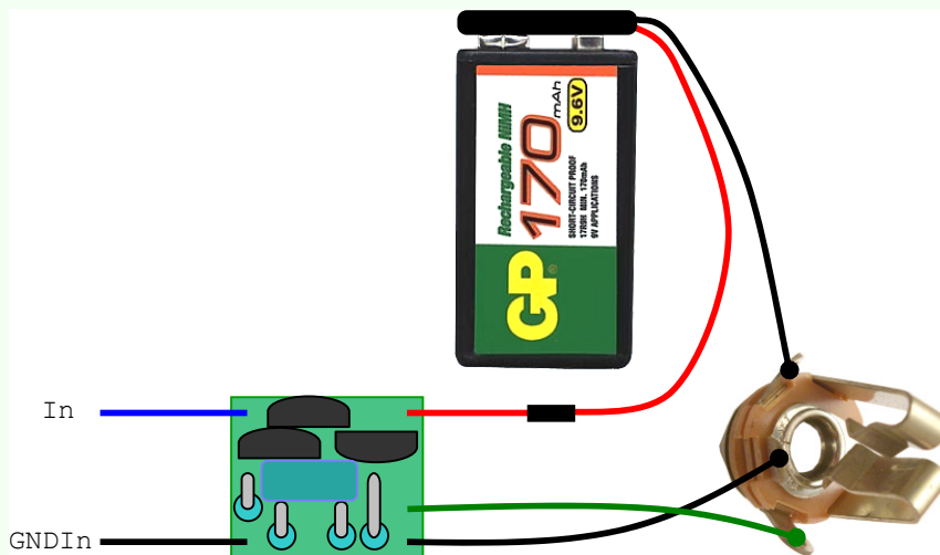
Abbildung 3-2: SB-1P-D2 direkt vor der Ausgangsbuchse
