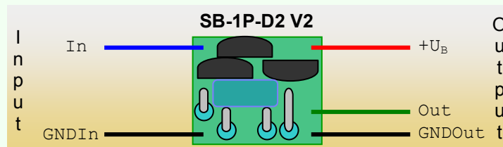
Abbildung 3-1: Die Platine des SB-1P-D2
